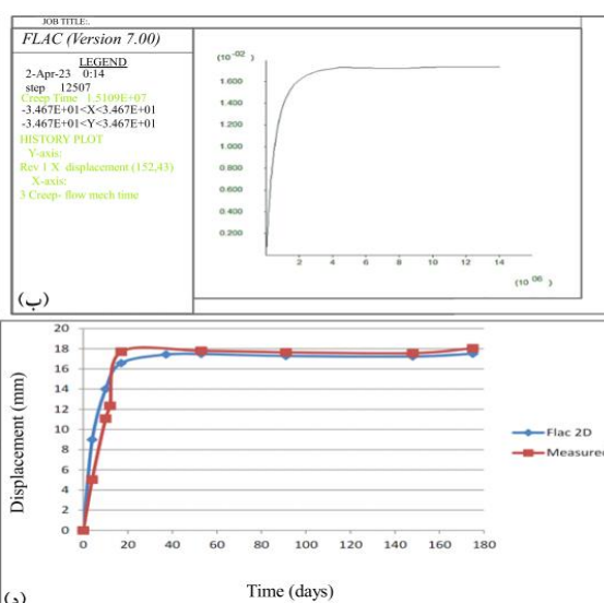
شکل ۷- (الف) منحنی مشخصه زمین، (ب) نمودار همگرایی به‌دست‌آمده از نرم‌افزار Flac2d در طول ۱۷۵ روز، (ج) منحنی‌های میزان جابه‌جایی در جهت افقی برای مقطع کیلومتر ۰+۶۹۰ تونل و (د) تطابق نتایج همگرایی ثبت‌شده توسط ابزار دقیق و به‌دست آمده از
