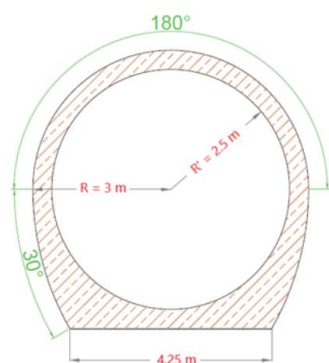
شکل ۲- ابعاد مقطع حفاری و مقطع نهایی تونل بعد از اعمال لاینینگ بتنی [۴۵]
