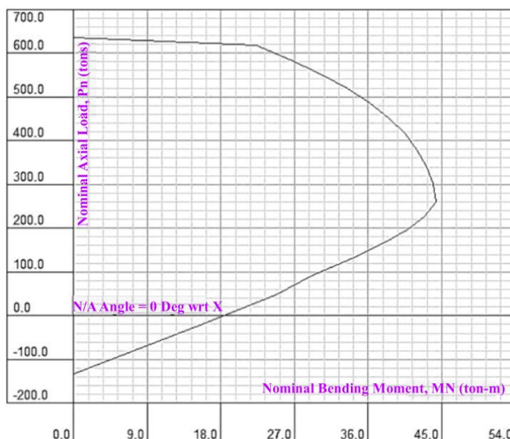
شکل ۹- دیاگرام ظرفیت مقطع پوشش نهایی تونل در نرم‌افزار Section Builder
