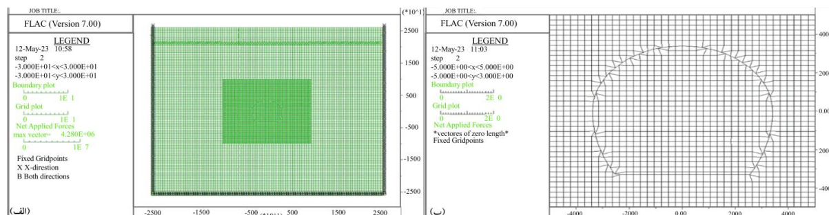
شکل ۴- (الف) مقطع مدل ایجادشده در نرم‌افزار Flac2D (کیلومتراژ ۰+۶۹۰) و (ب) مقطع حفاری تونل ایجادشده نرم‌افزار Flac2D
