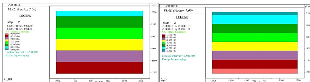
شکل ۸- (الف) منحنی‌های میزان تنش قائم مقطع ۰+۶۹۰ و (ب) منحنی‌های میزان تنش افقی مقطع ۰+۶۹۰
