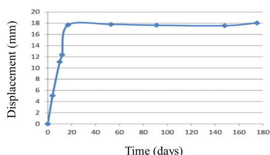
شکل ۶- نتایج همگرایی ثبت‌شده برای تونل در طول ۱۷۵ روز در مقطع ۰+۶۹۰
