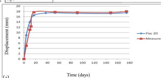
شکل ۷- (الف) منحنی مشخصه زمین، (ب) نمودار همگرایی به‌دست‌آمده از نرم‌افزار Flac2d در طول ۱۷۵ روز، (ج) منحنی‌های میزان جابه‌جایی در جهت افقی برای مقطع کیلومتر ۰+۶۹۰ تونل و (د) تطابق نتایج همگرایی ثبت‌شده توسط ابزار دقیق و به‌دست آمده از
