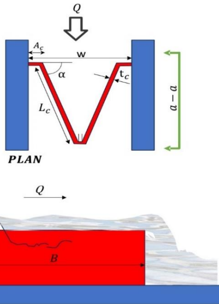
شکل ۲- شماتیک هندسه سرریز نوک اردکی به همراه مدل آزمایشگاهی
