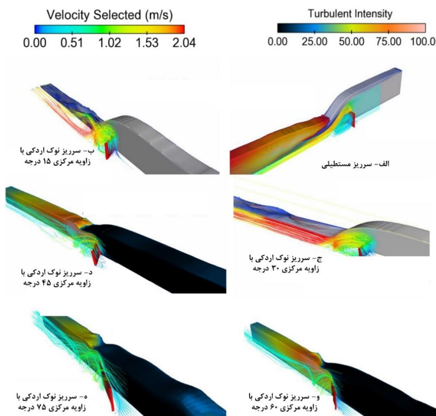
شکل ۱۶- الگوی سرعت جریان و شدت آشفتگی بر روی سرریزهای نوک اردکی به ازای زوایای بازشدگی مختلف
