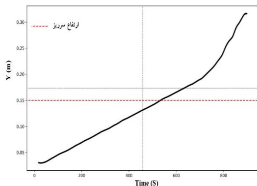
شکل ۵- شرایط مرزی پایین‌دست سرریز نوک اردکی در حالت مستغرق
