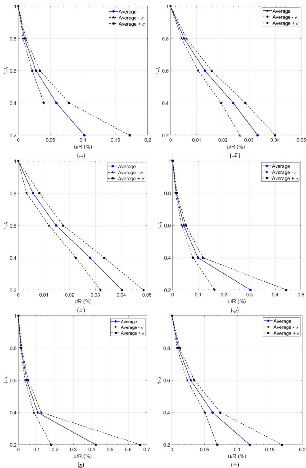
شکل ۵- منحنی مشخصه زمین به ازای (الف) D = 8 \text{ m} و z = 20 \text{ m} ، (ب) D = 8 \text{ m} و z = 40 \text{ m} ، (پ) D = 8 \text{ m} و z = 60 \text{ m} ، (ت) D = 12 \text{ m} و z = 20 \text{ m} ، (ث) D = 12 \text{ m} و z = 40 \text{ m} ، (ج) D = 12 \text{ m} و z = 60 \text{ m}
