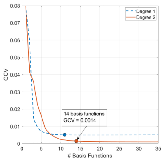
شکل ۸- تغییرات GCV با تعداد توابع پایه
